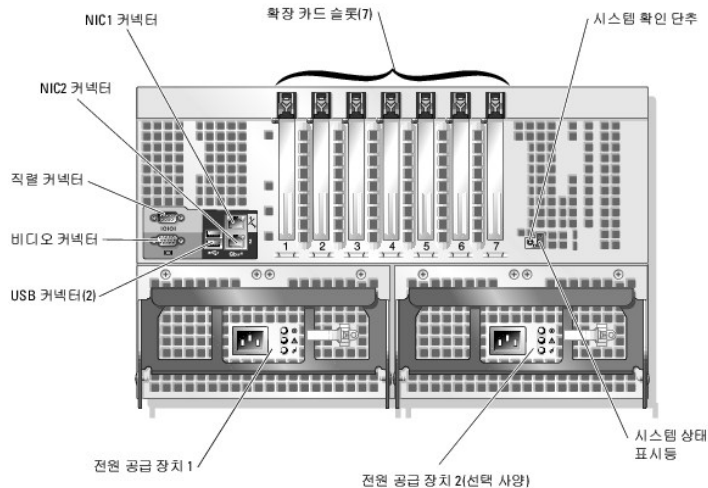
그림 1-4. 후면 패널 구조 및 표시등
