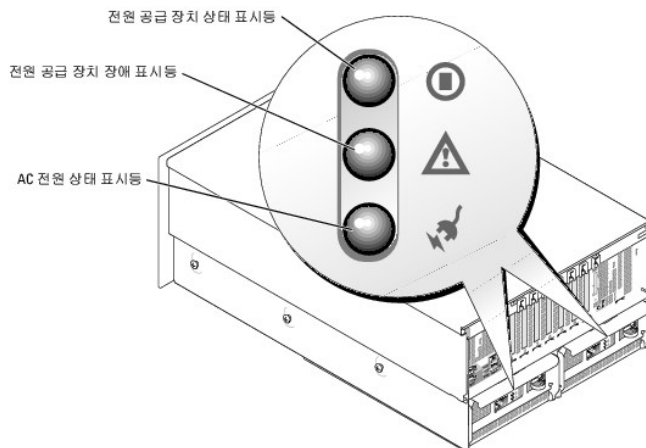
그림 1-5. 전원 공급 장치 표시등
