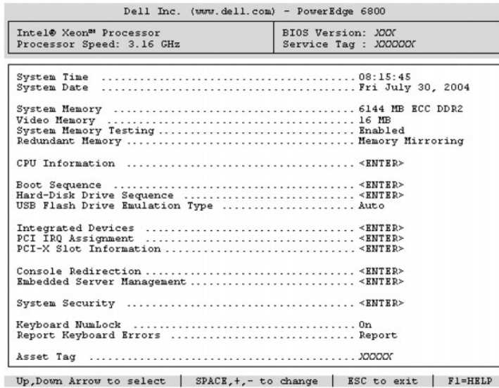
그림 3-1. System Setup 프로그램 기본 화면
